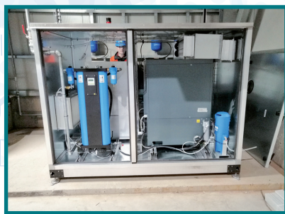
Modulo con compressore e sistema di termoregolazione per funzionamento con temperatura ambiente di -30^{\circ}\text{C} , installato in POLONIA.
