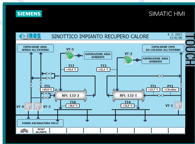
Quadro di comando con PLC che gestisce il funzionamento in automatico del sistema di recupero.
